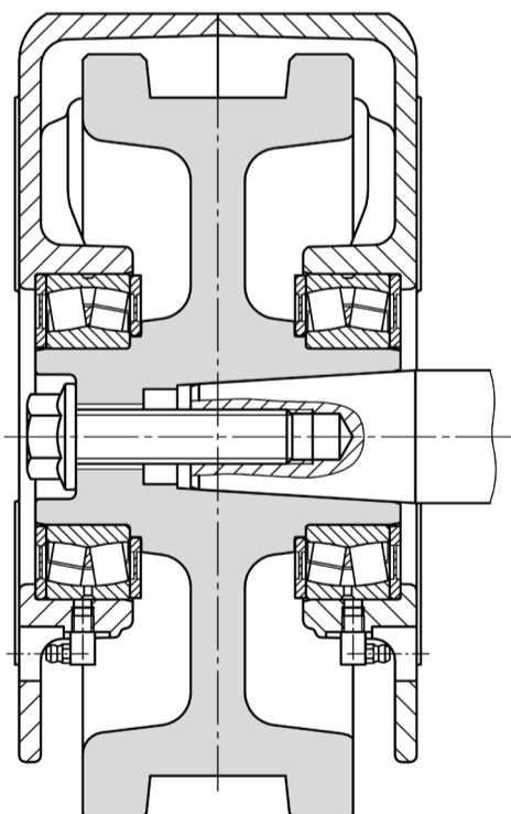
Bloque de ruedas accionado
