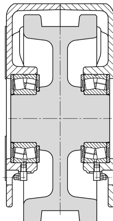
Bloque de ruedas no accionado
