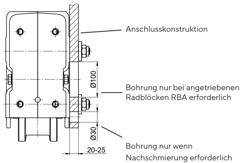
Schnittansicht
