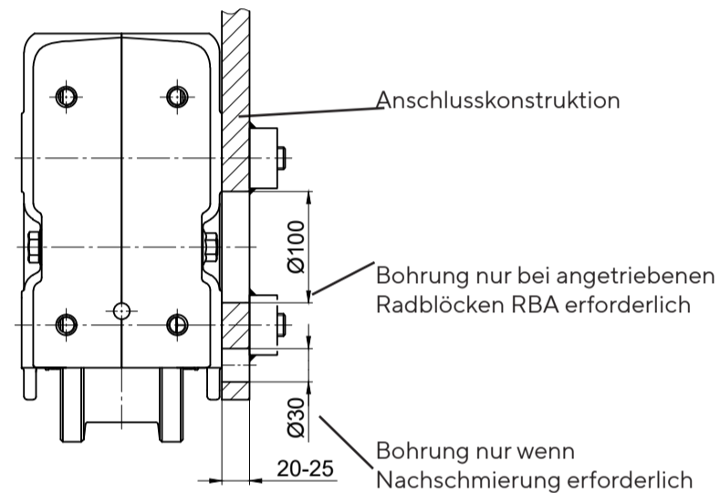
Schnittansicht
